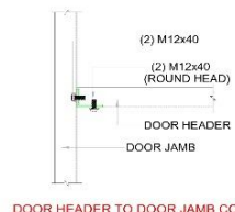
DOOR HEADER TO DOOR JAMB CONN. DETAIL
